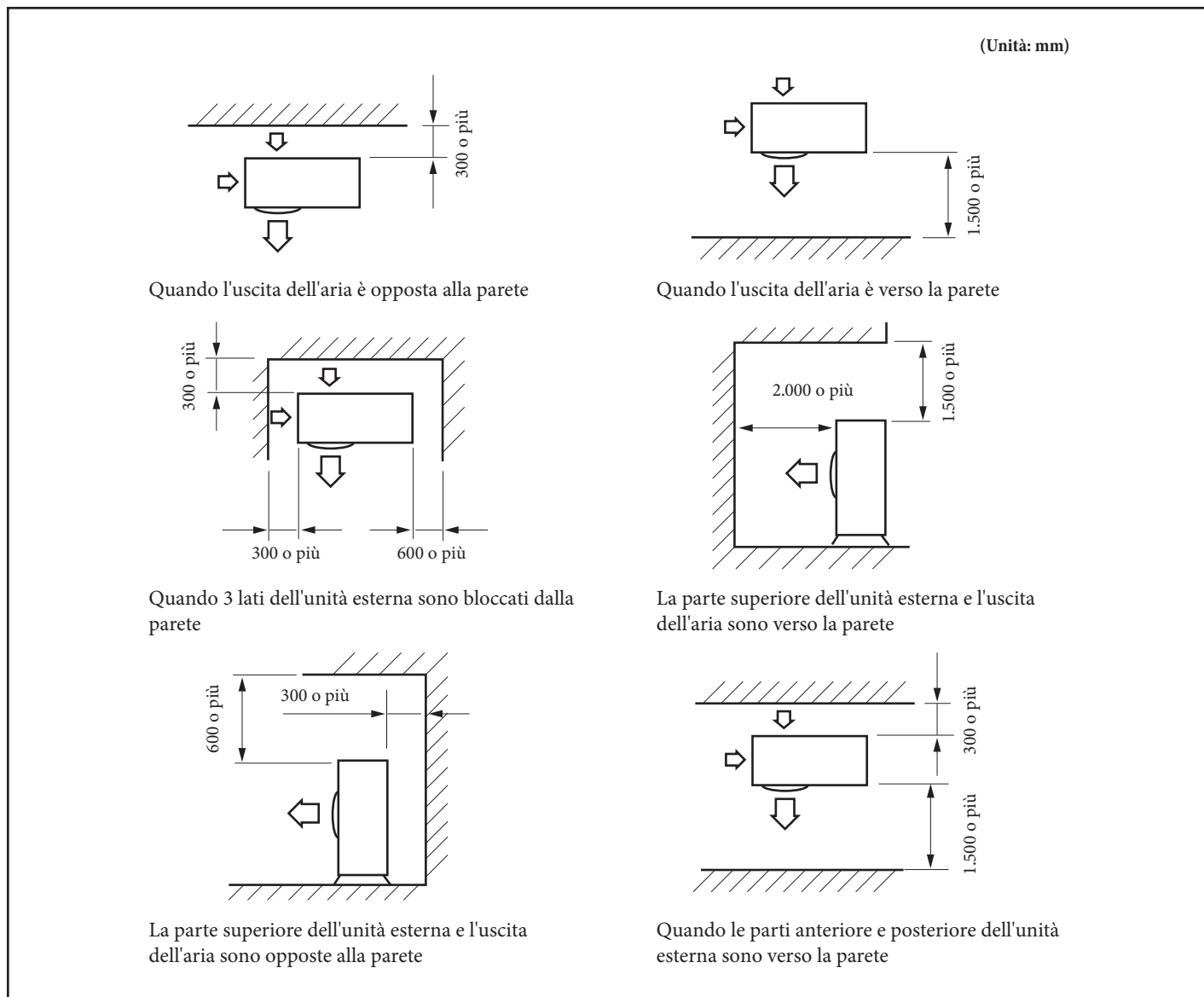
4.11 REQUISITI DI SPAZIO PER L'UNITA' ESTERNA. Installazione di un'unità esterna singola
